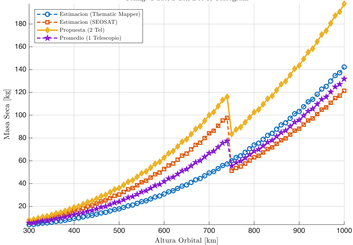
Comparativa de Masa Seca vs. Altura Config: 2 Sat, 2 Tel, Det 1, Cassegrain
